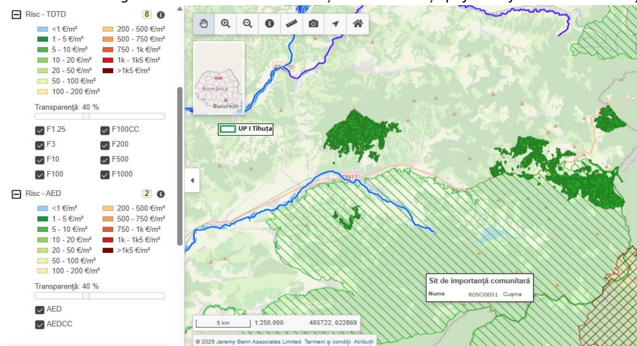
* Fig. 3.1.10.1.2.. Hartă de hazard și risc la inundații pt fondul forestier U.P. I Tihuța
