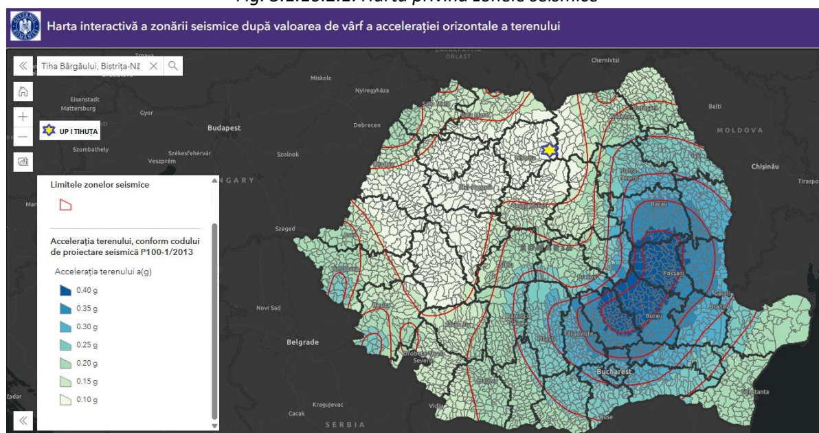
Fig. 3.1.10.2.1. Harta privind zonele seismice
