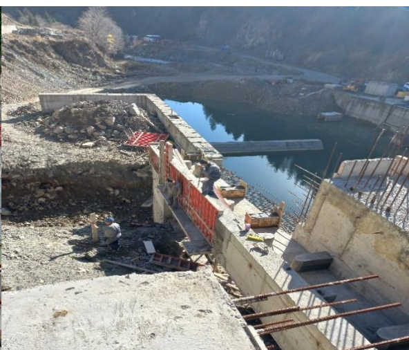
Foto nr. 4 – Scară de pești-cofrare
