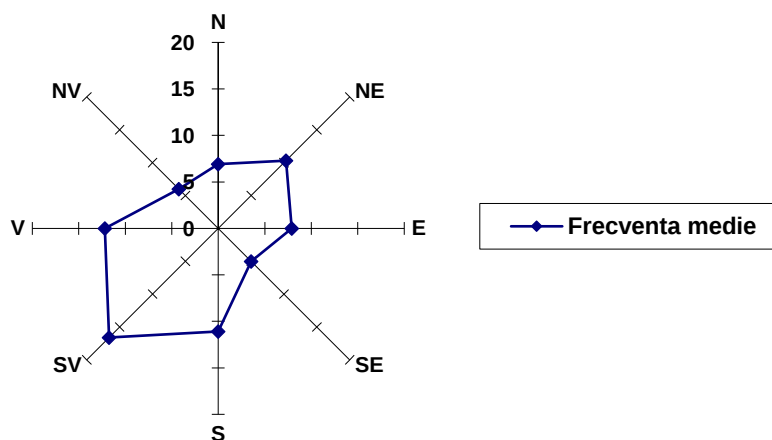
Graficul vitezei medii anuale a vanturilor
