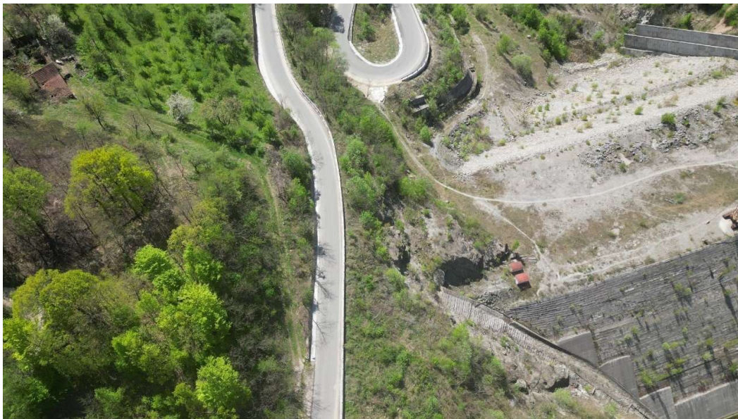
Figura nr. 81 – Imagine aeriană cu flancul stâng al barajului Cornereva, acolo unde este ancorat în versantul corespunzător, în conglomeratele cuarțitice ale Formațiunii de Gresten. Vegetația de aici, pionieră, nu este considerată a reprezenta habitate N2000
