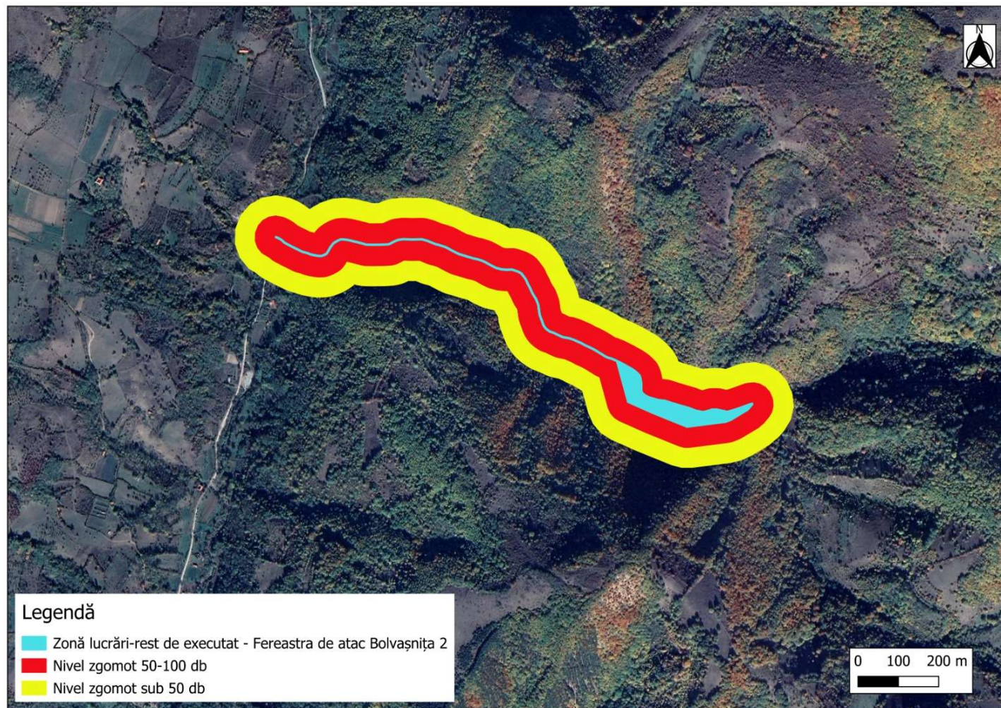
Figura nr. 54.3 Dispersia zgomotului din zonele cu lucrări – zona Bolvașnița II
