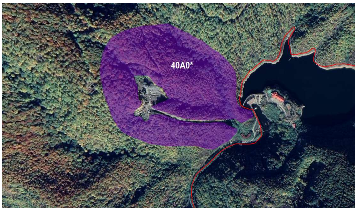
Figura nr. 114 – Harta habitatelor neforestiere din perimetrul castelului de echilibru, nodului de presiune și conductei forțate de pe versantul drept al Cernei
