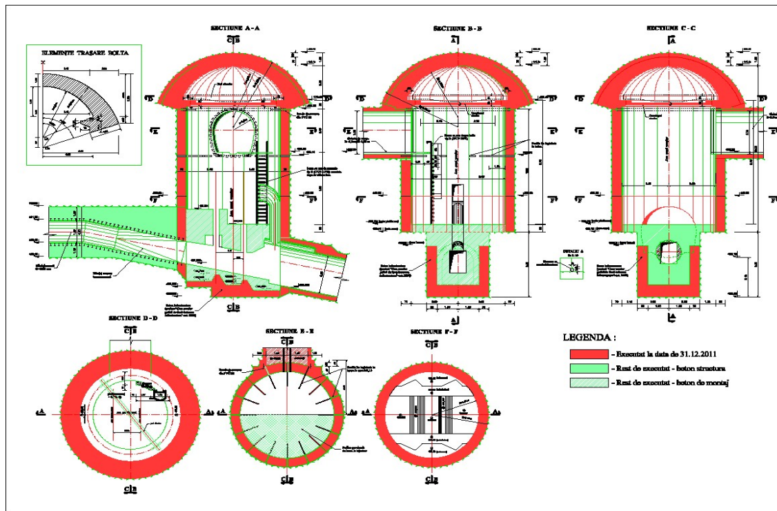
Figura nr. 42 Casa vanelor golirii de fund
