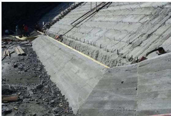
Figura nr. 21 Vatra barajului. Zona din albic versant stâng
