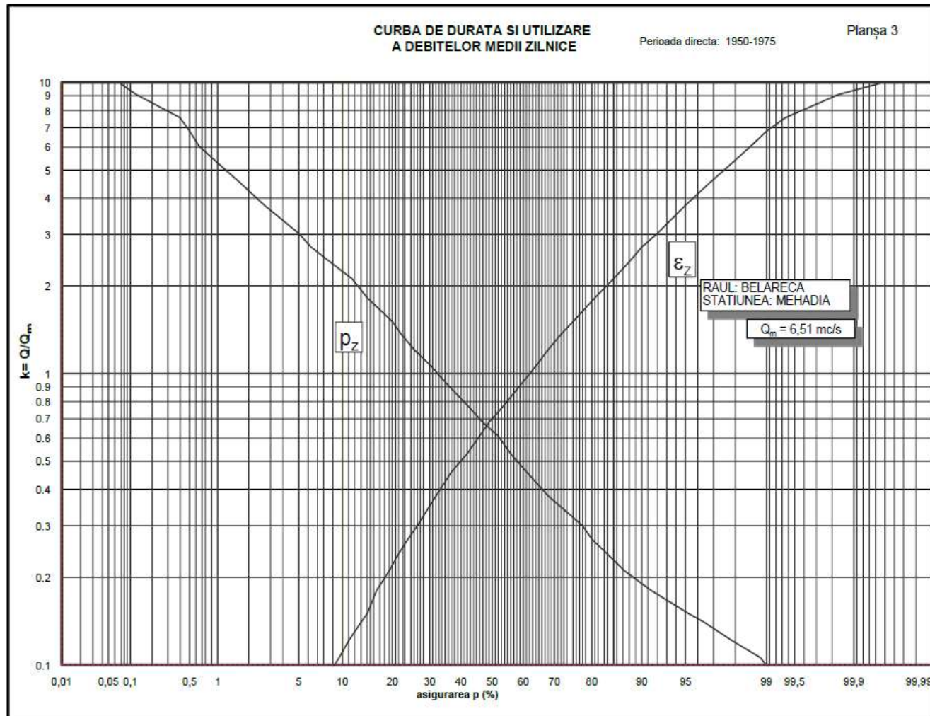
Figura nr. 15 Curba de durată și utilizare a debitelor medii zilnice – R. Belareca
