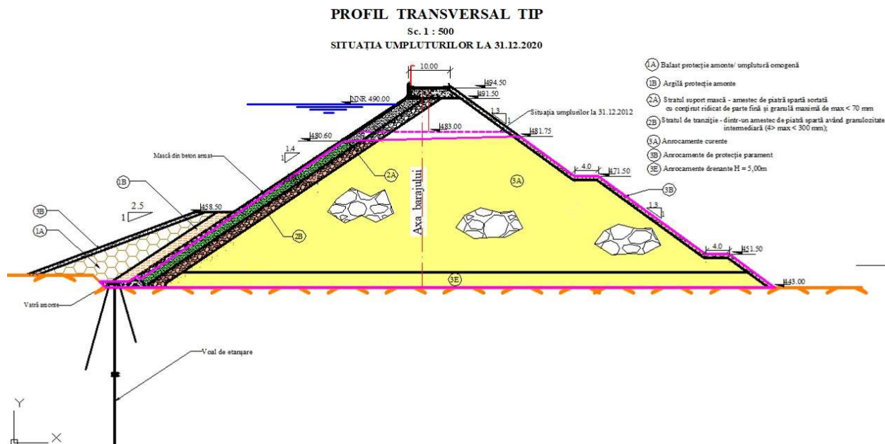
Figura nr. 20 - Profil transversal tip baraj. Situația umpluturilor la 31.12.2020
