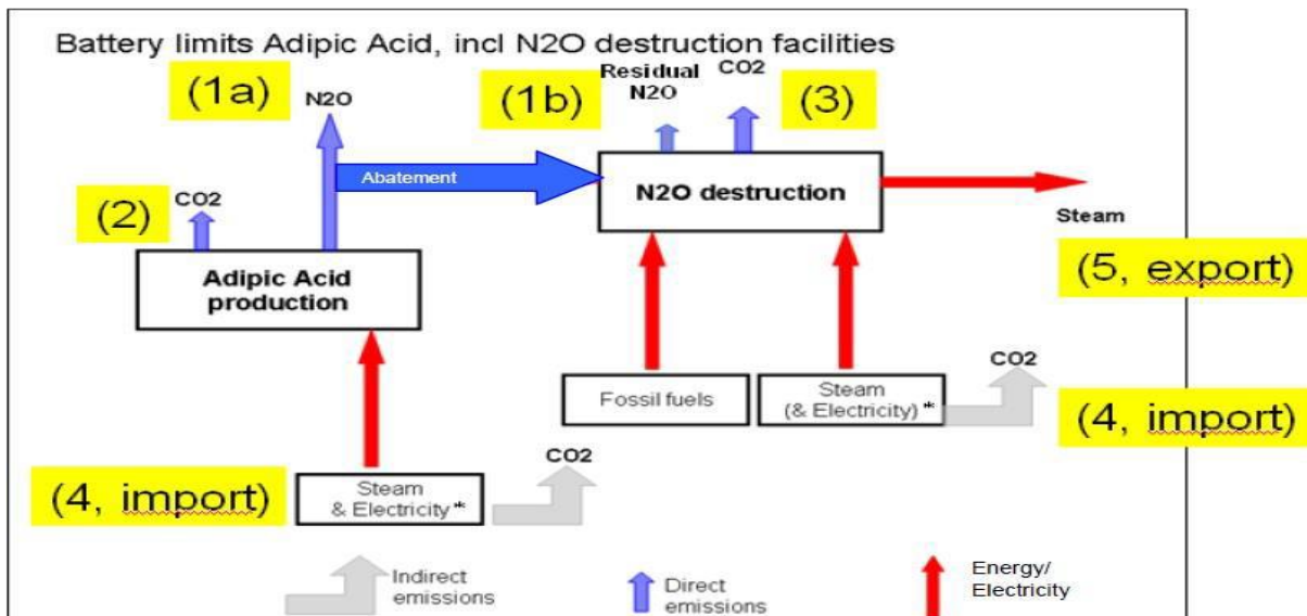
Figura 6. Emisiile incluse în indicatorul de referință a produsului pentru acidul adipic (emisiile definite prin câmpul galben sunt acoperite; descrierile acelor câmpuri sunt furnizate în text (Regulament pentru acidul adipic, 2010);
