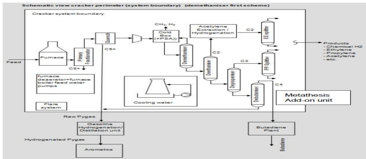
Figura 8. Limitele sistemului pentru indicatorul de referință cracarea cu abur (Norme pentru cracarea la abur, 2010)
