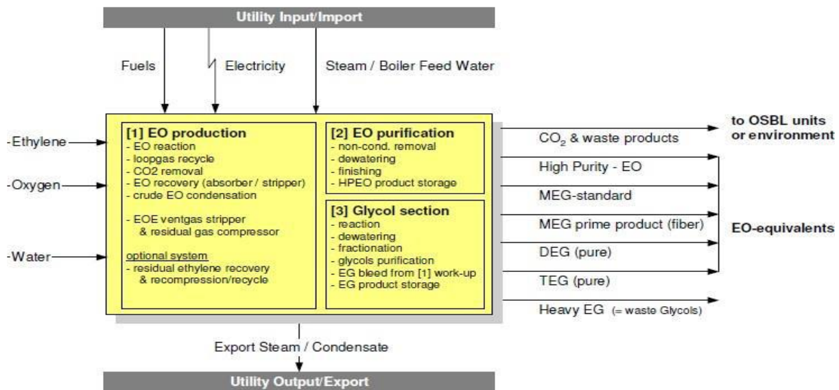
Figura 9: Intrări și ieșiri ale unităților EO și EG incluse în indicatorul de referință. (PDC (2010), Norme pentru sectorul oxid de etilenă și derivații acestuia)
