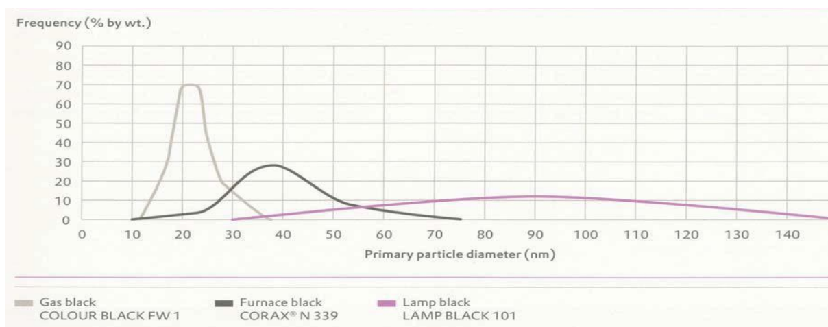
Figura 5. Diametrul particulelor primare din negrul de fum (Regulament pentru negrul de fum, 2010)
