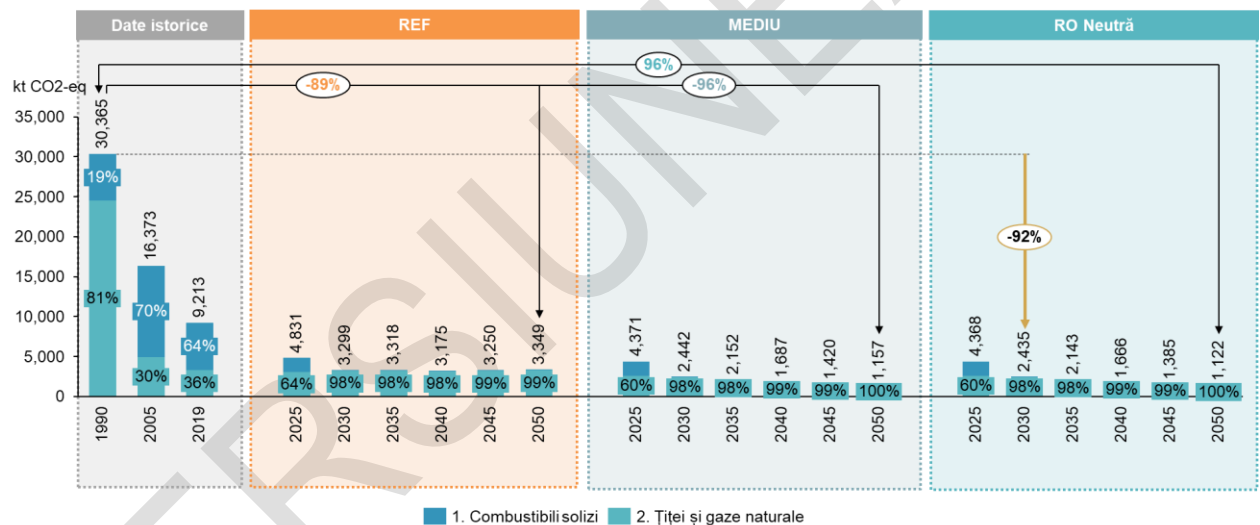
Figura 32. Evoluția emisiilor fugitive produse de combustibili conform celor 3 scenarii analizate: REF, Mediu și RO Neutră
